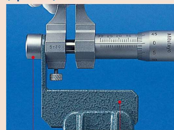
Cap (300401)
